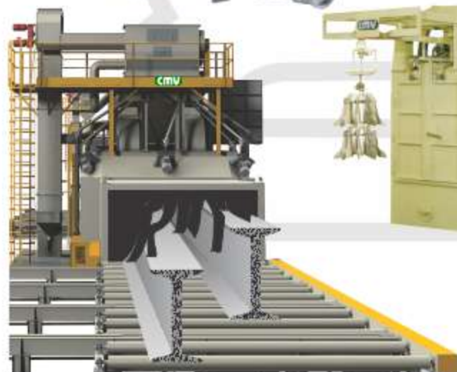
Granalladora con Transportador de Rodillos para Placas y Perfiles Roller Conveyor Shot Blast Machine
